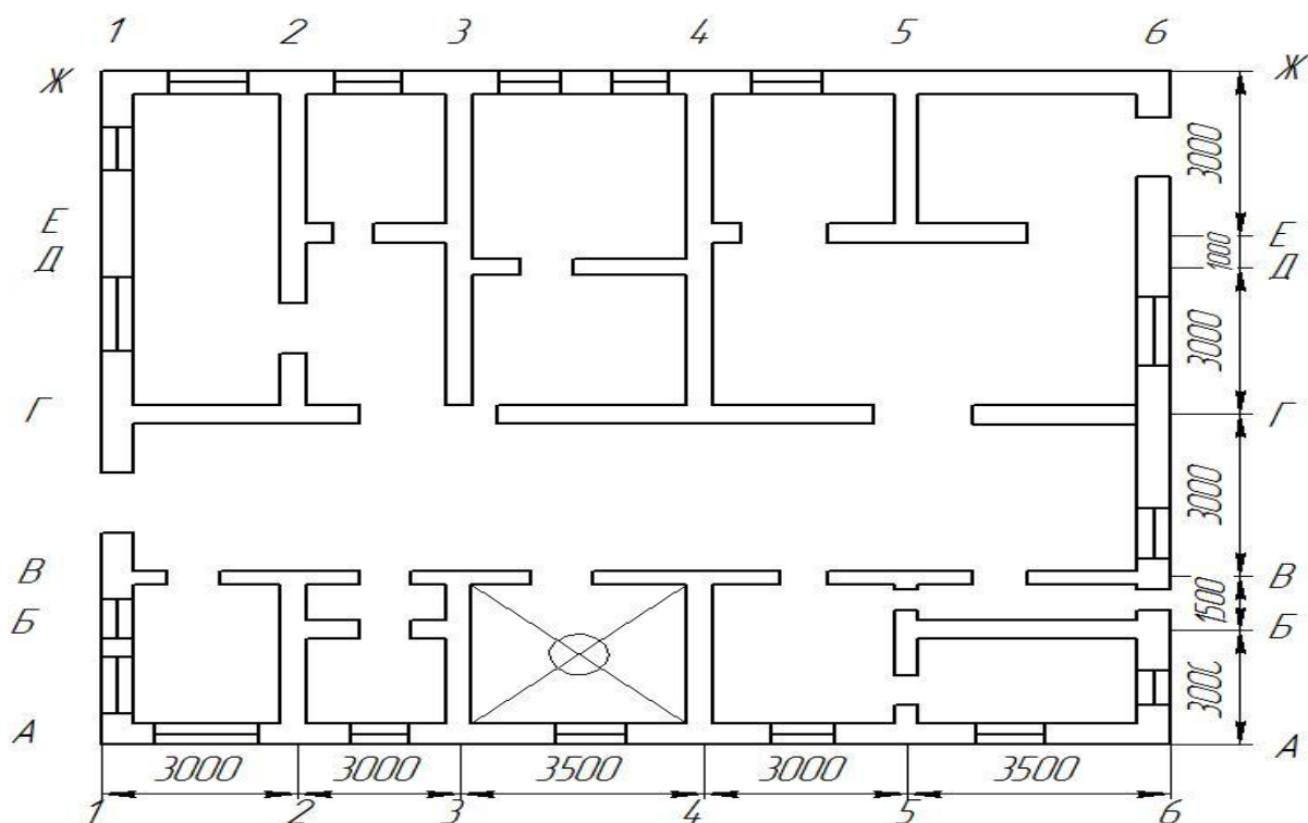
Рисунок 1 – План здания
