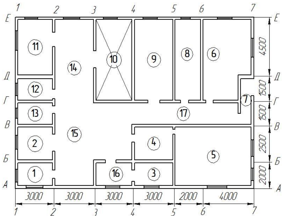
Рисунок 1 –План здания
