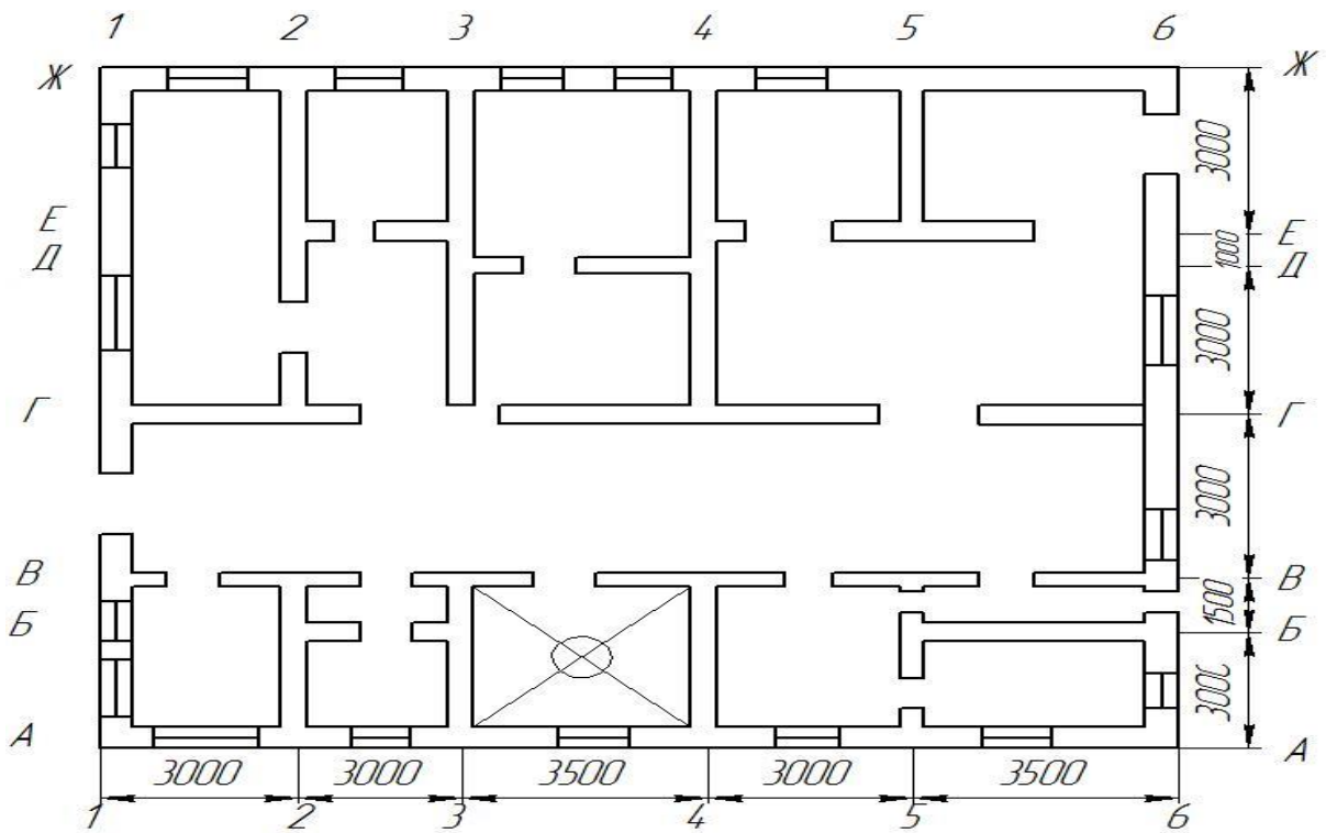
Рисунок 1 - План здания
